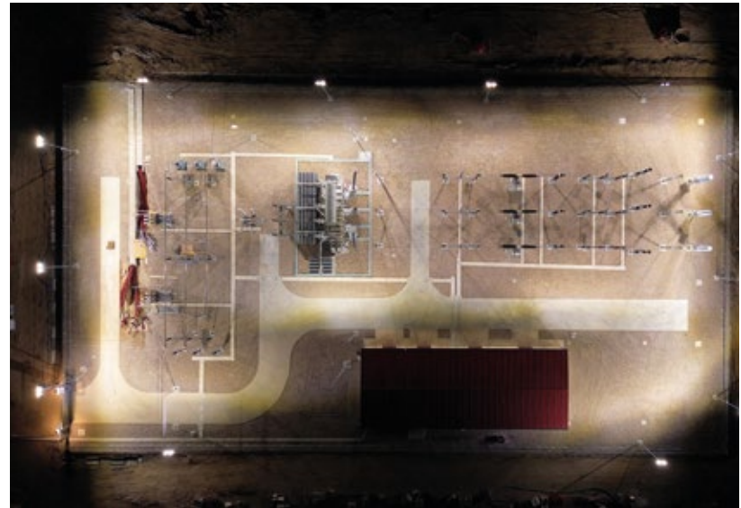
△ SET Husillos 400/132, líneas aérea y subterránea AT de evacuación (Palencia)
