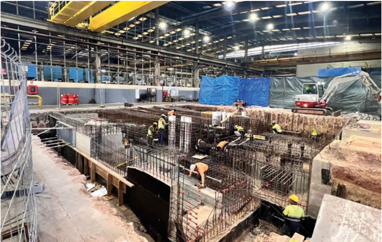
▼ Laminador en frío nº2 en Segorbe (Castellón)
