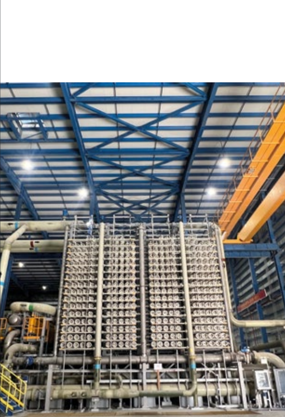
▲ Desaladora Jubail 3A (Arabia Saudí)
